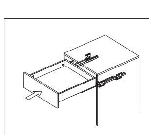
Szuflada zamyka się cicho dzięki zintegrowanemu systemowi cichego domyku
