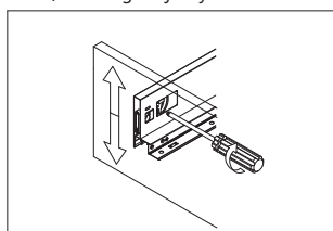
Montaż ścianki tylnej szuflady
