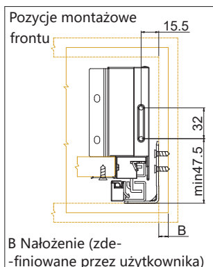
Pozycja łączników frontu
