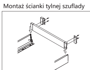
Montaż szuflady
