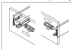
Montaż dna szuflady
