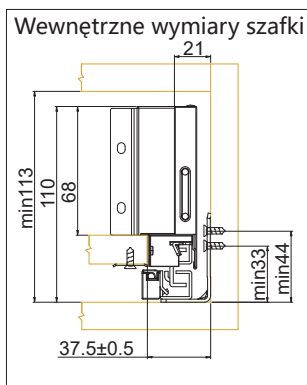
Wewnętrzne wymiary szafki
