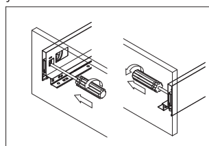
Montaż frontu szuflady
